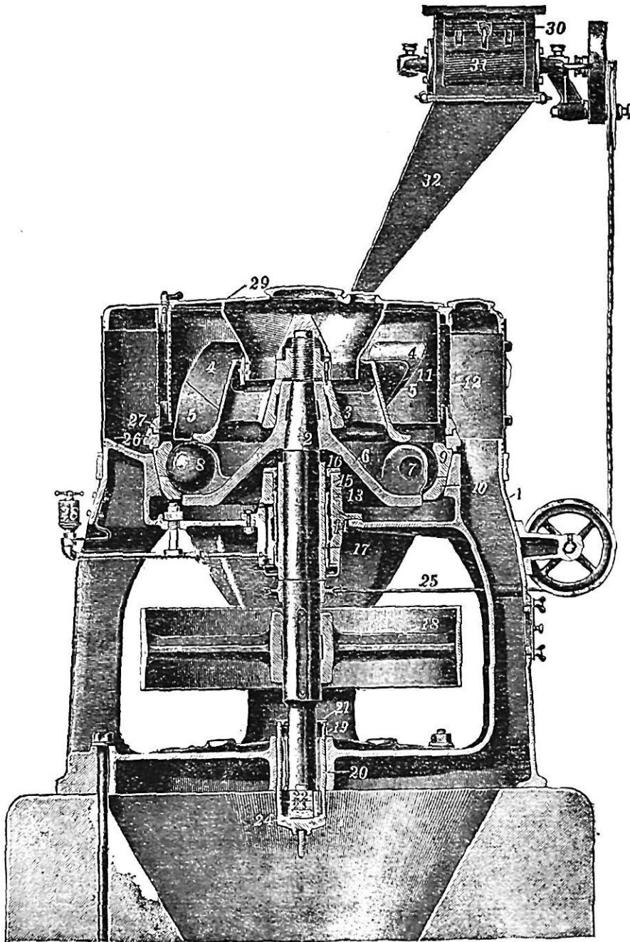
FIG. 16.—The Roulette Mill.
