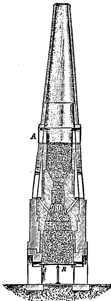
FIG. 27.—Aalborg Kiln.
