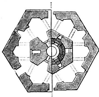
FIG. 2.—Rüdersdorf Kiln.
