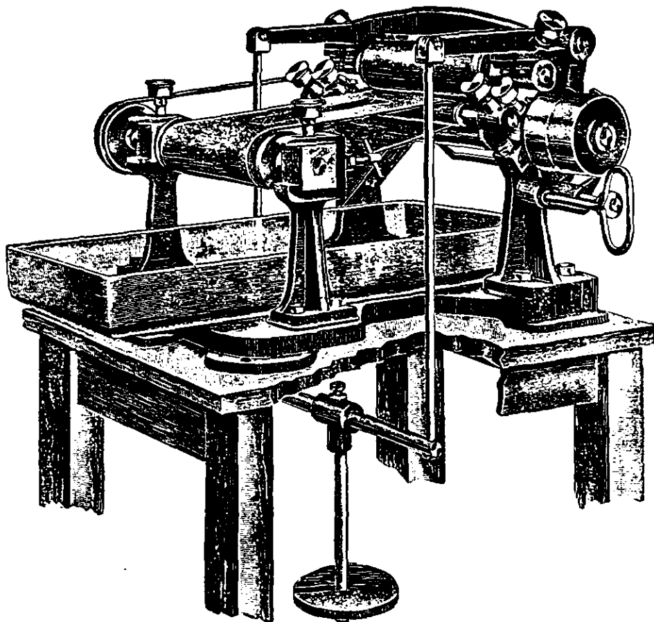
FIG. 14.—Impregnating Machine, \frac{1}{10} Actual Size.
