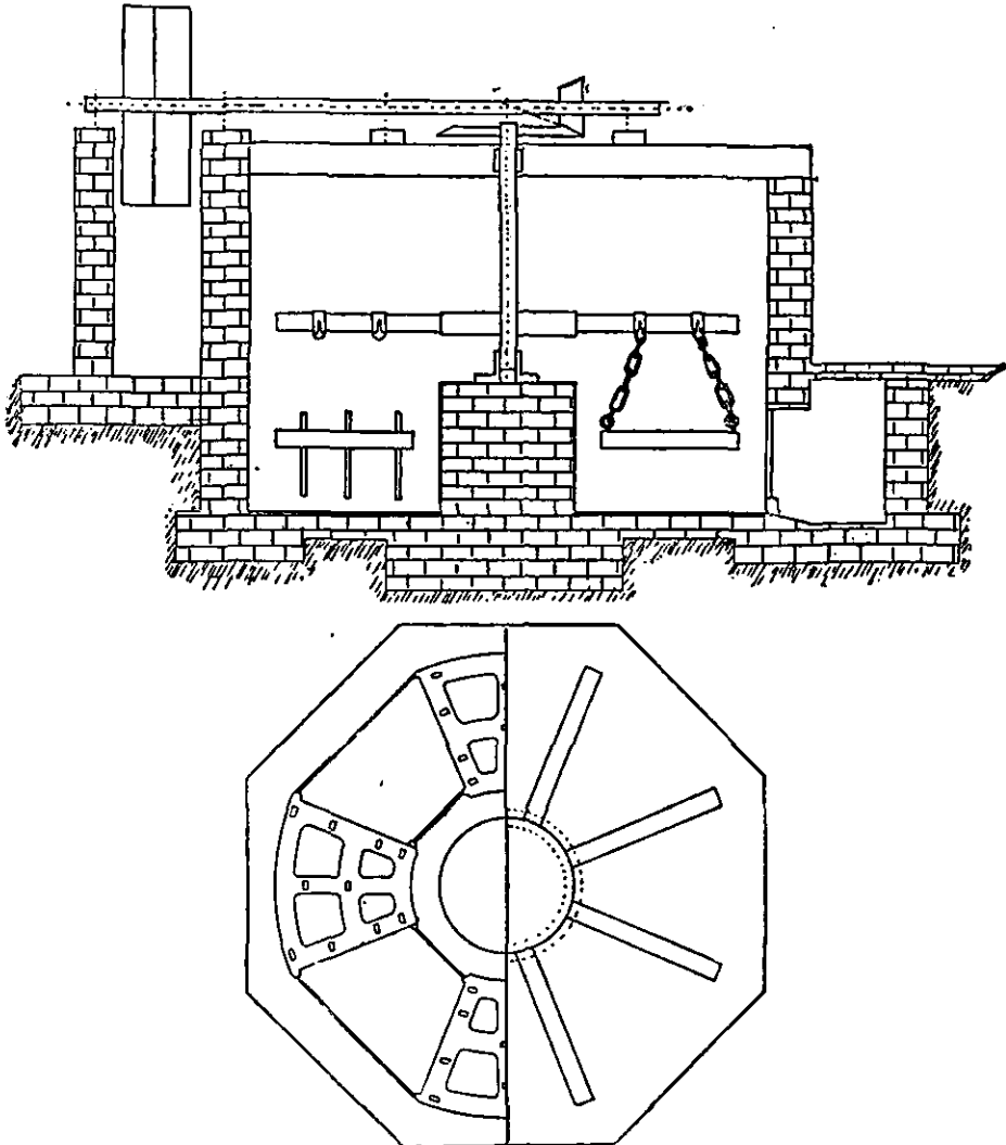
FIG. 7.—Wash Mill.
