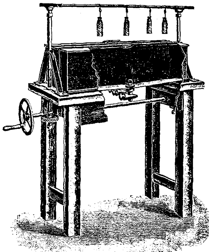
FIG. 18.—Collodionising Bath, \frac{1}{8} Actual Size.
