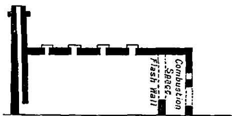
FIG. 18.—Newcastle or Horizontal Kiln.
