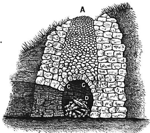
FIG. 1.—Intermittent Kiln.
