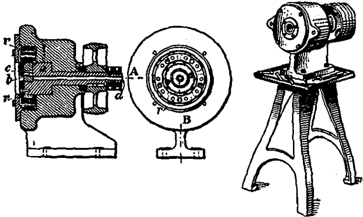
FIG. 13.—Section on A. B.
