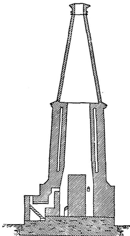
FIG. 3.—Fahnehgelm Kiln.
