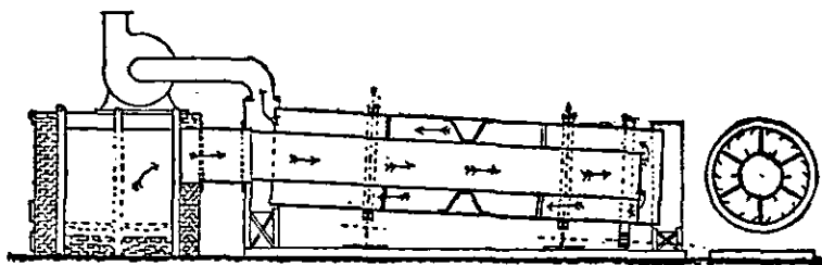
FIG. 5.—Ruggles-Coles Drier.
