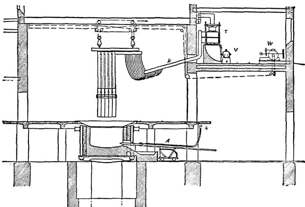
FIG. 10. -Modern Carbide Plant.
