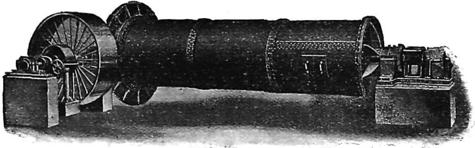
FIG. 4.—Tube Mill. (Edgar Allen & Co. Ltd., Sheffield.)
