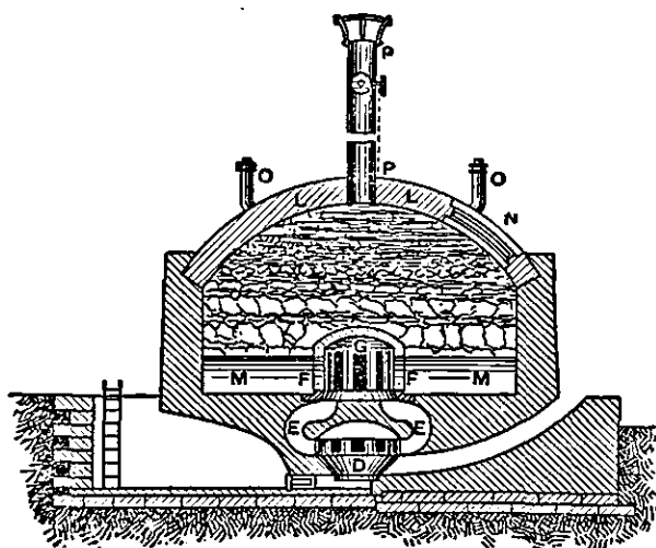
FIG. 30.—Dumesnil Kiln.
