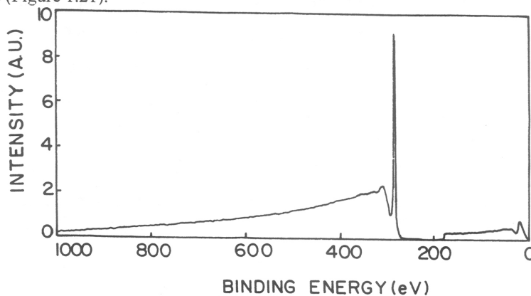
Figure1.19: XPS spectrum of PE
